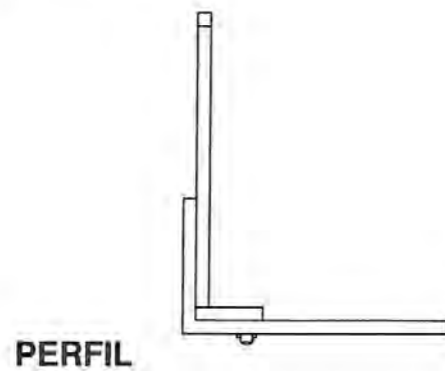
PASO PEATONAL SOBRE ZANJA EN CALZADA DESPIECE PASARELA TIPO Cotas en mm.
