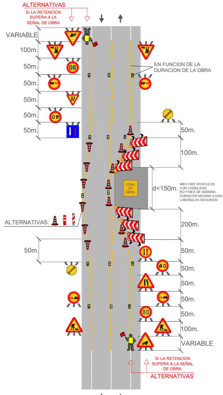
EJEMPLO: 1.11 VIA DE DOBLE SENTIDO DE CIRCULACIÓN, CALZADA UNICA CON DOS CARRILES
