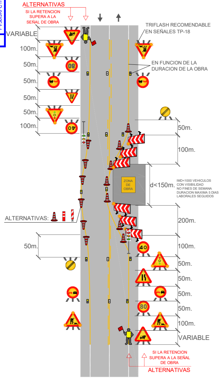
EJEMPLO: 1.13 VIA DE DOBLE SENTIDO DE CIRCULACIÓN, CALZADA UNICA CON DOS CARRILES
