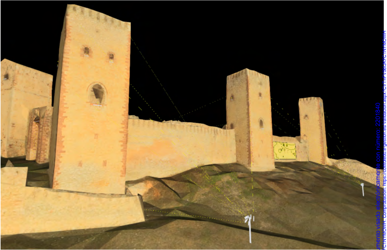
APUNTAMIENTO_Alzado Sur
