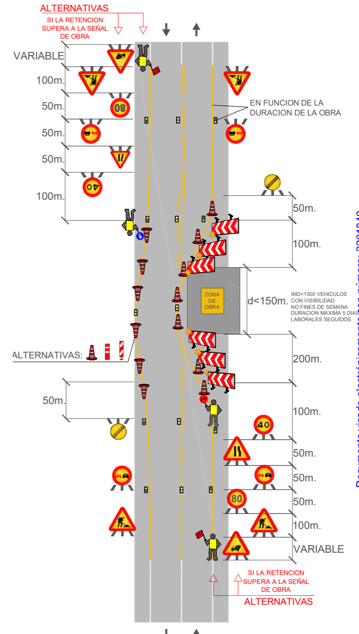
EJEMPLO: 1.12 VIA DE DOBLE SENTIDO DE CIRCULACIÓN, CALZADA UNICA CON DOS CARRILES
