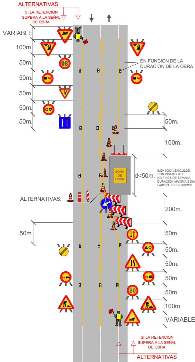
EJEMPLO: 1.6 VIA DE DOBLE SENTIDO DE CIRCULACIÓN, CALZADA UNICA CON DOS CARRILES
