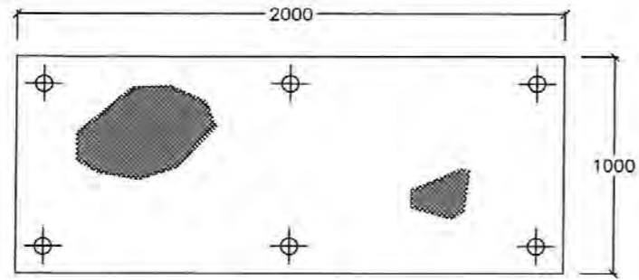
PISO CHAPA DE ACERO ANTIDESLIZANTE e=5 mm.
