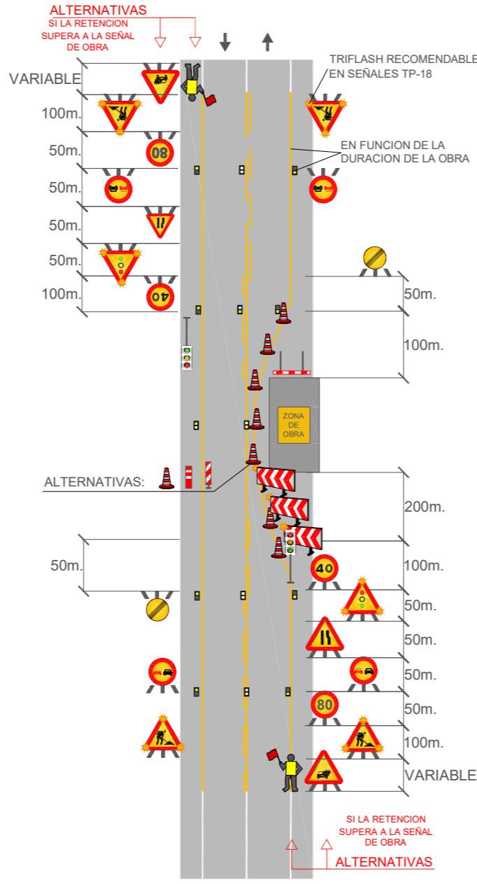
EJEMPLO: 1.8 VIA DE DOBLE SENTIDO DE CIRCULACIÓN, CALZADA UNICA CON DOS CARRILES
