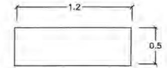
PLANCHA TIPO. MADERA PINTADA EN COLOR AMARILLO DE SEÑALIZACIÓN Y PERFILES DE CHAPA GALVANIZADA
